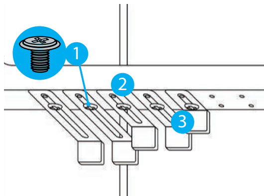
Rysunek 3.8.1.1. Obudowa SC01-4504-10B i SC01-5504-10B
