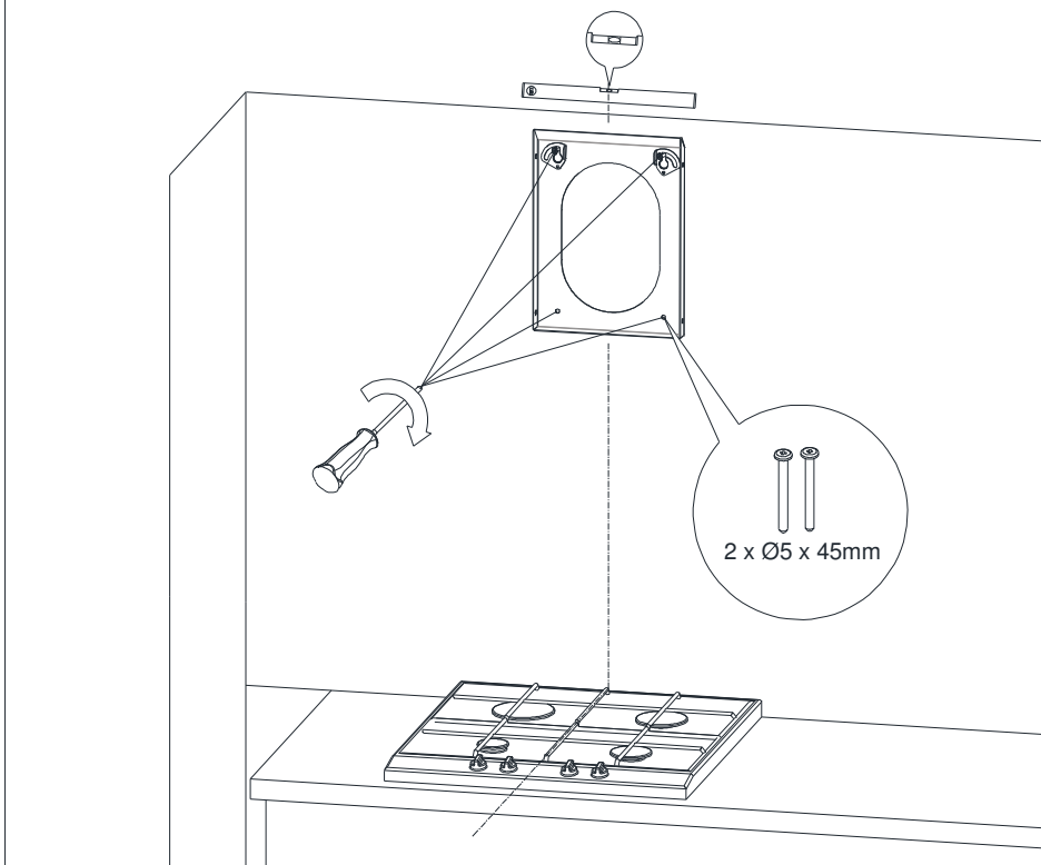
Rys. 9 Ustawienie uchwyty mocowania okapu.
