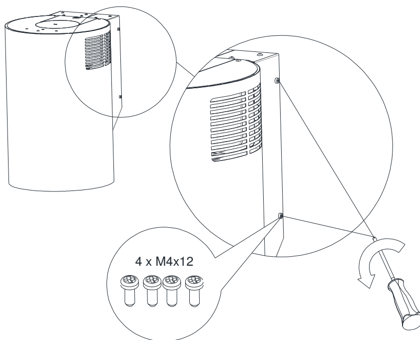
Rys. 7 Demontaż uchwytu mocowania okapu.
