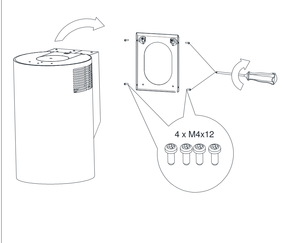
Rys. 10 Montaż okapu na uchwycie ściennym.
