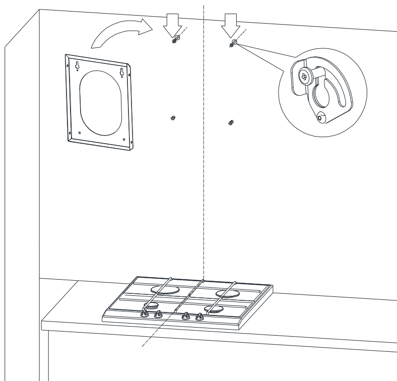
Rys. 8 Zawieszanie uchwytu mocowania okapu.
