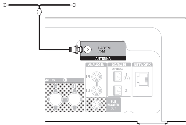
Pokojowa antena DAB/FM (w komplecie)
