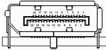
20-pinowy kabel sygnałowy kolorowego wyświetlacza
