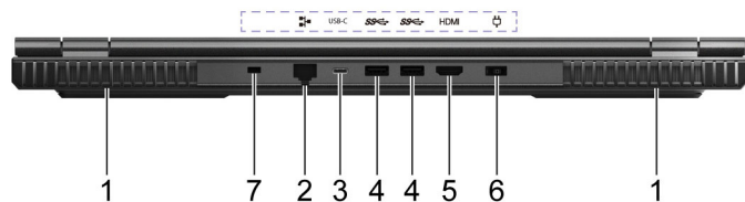
Rysunek 8. Widok z tyłu - modele 17-calowe
