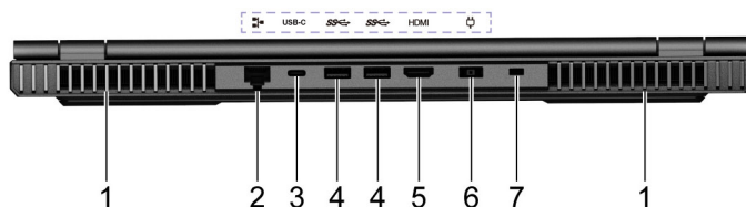
Rysunek 7. Widok z tyłu - modele 15-calowe
