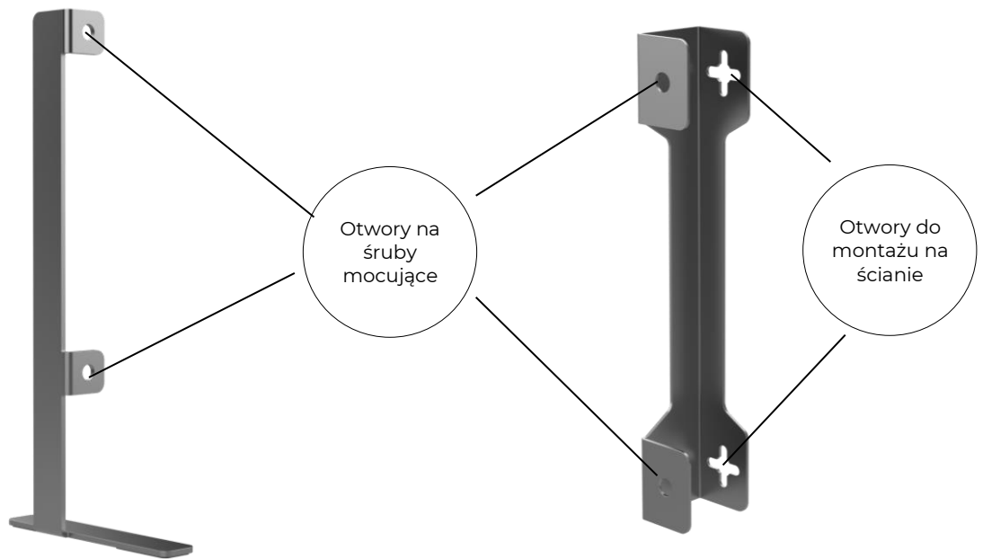
Nóżka do montażu na podłodze*
