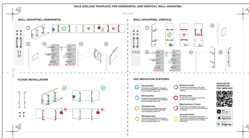
Szablon do wiercenia otworów w ścianie
