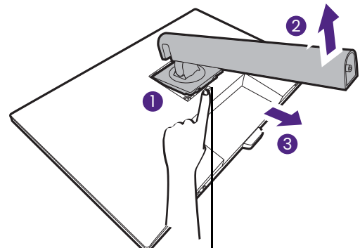
Przycisk zwalniania
