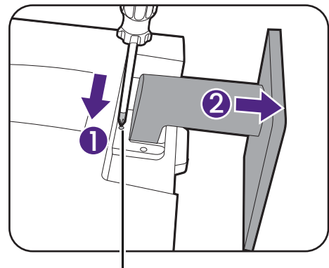
Przycisk zwalniania
