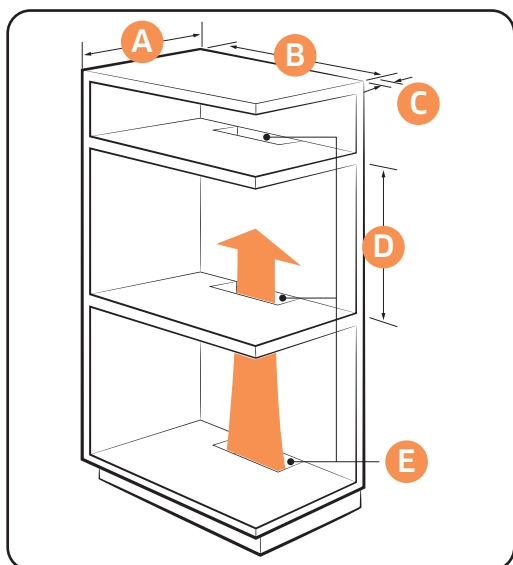
Szafka do zabudowy (mm)
