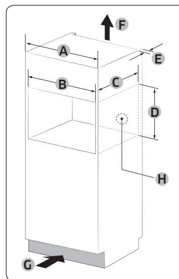
Szafka do zabudowy (mm)
